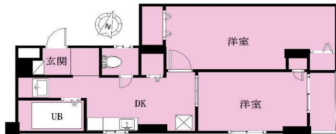
平面図
